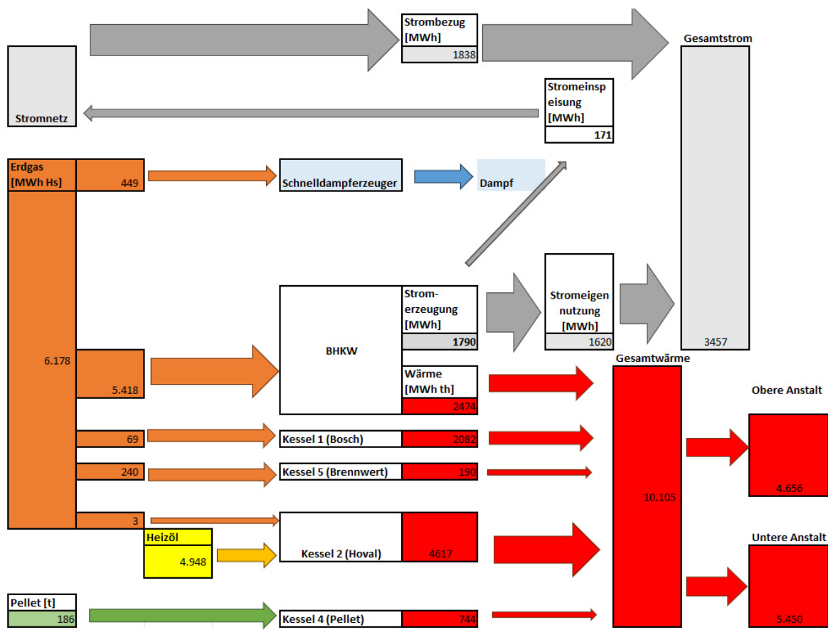
Energieflussdiagramm Standort Bayreuth
